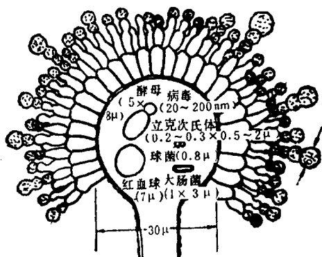
图 1-1 微生物大小的比较
