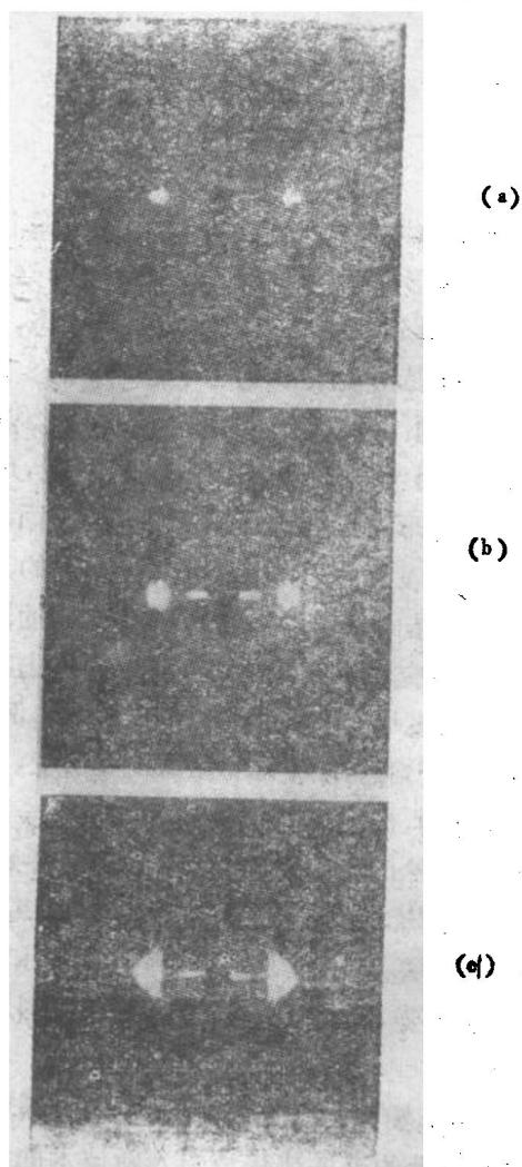
图 1.1 三个拉伸的聚乙烯的广角X射线衍射图。除了很多尖锐的取向结晶反射外,还应注意那未取向的“无定形”的弥散环。在分子量很大的聚合物中(b)和支化的聚合物中(c),弥散环比典型的商品线形聚合物(a)的强得多
