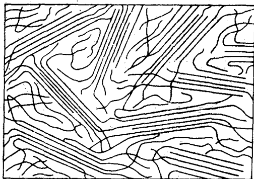
图 1.2 聚合物结构的缨状胶束模型(见Bunn, 1953)
