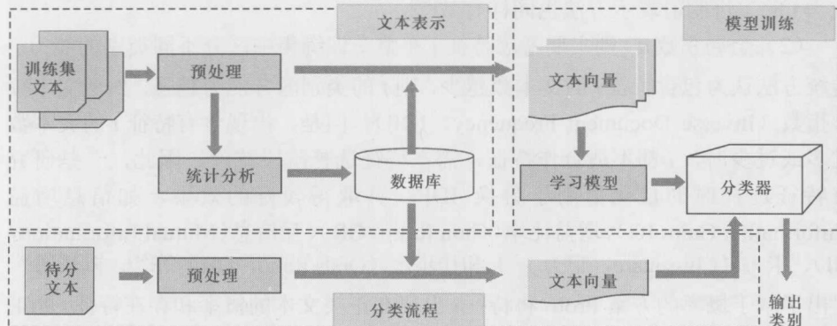
图 1-1 文本分类模型
