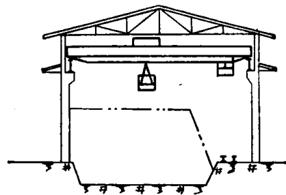
图1—1—2 半地下式矿仓
