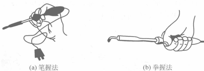
图 1.1.6 电烙铁的握法
