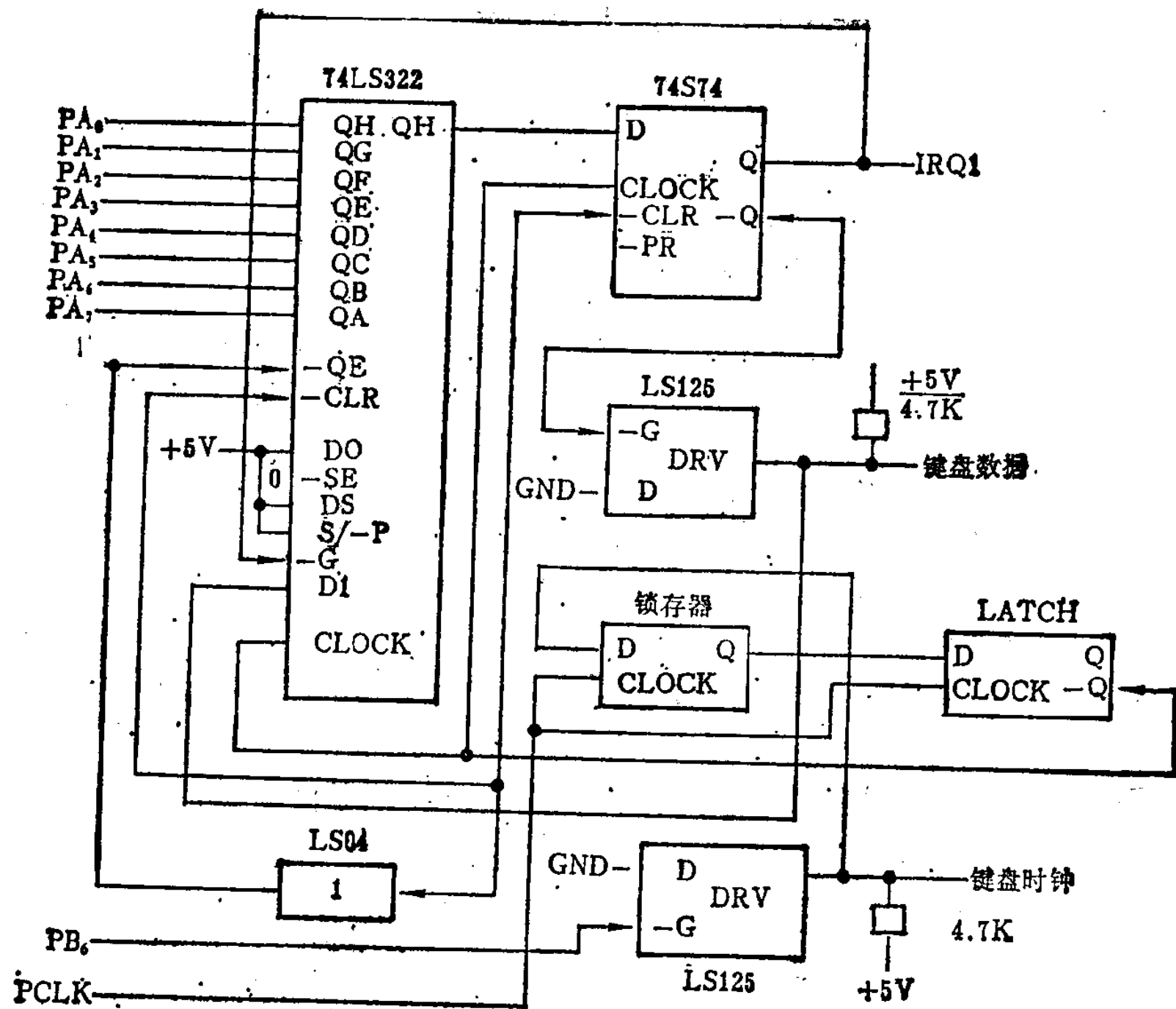
图 18-2 键盘接口框图
