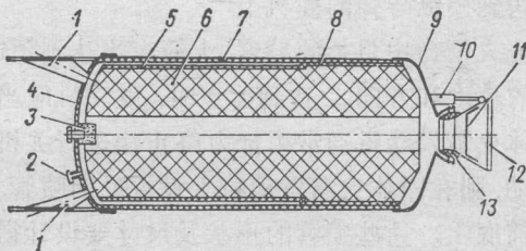
图 1.2 固体火箭发动机的结构示意图
