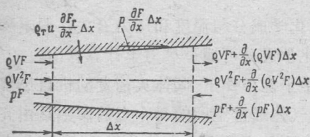
图 2.1 运动方程组的推导
