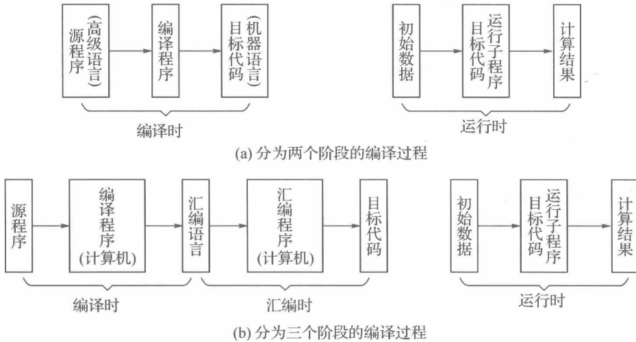
图 1.1 编译过程
