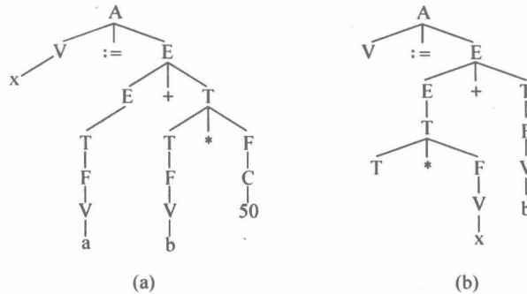
图 1.4 语法树
