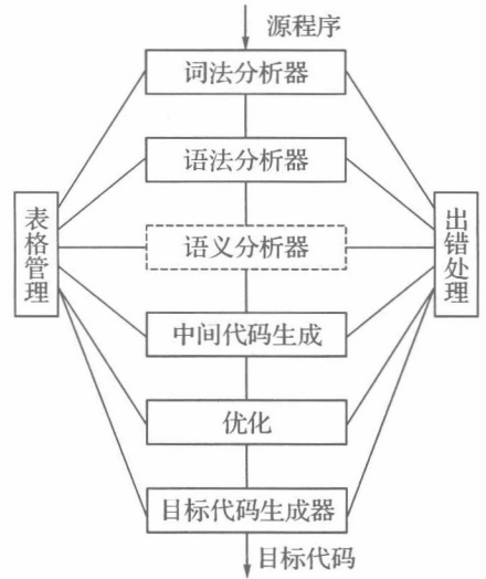
图 1.3 编译阶段
