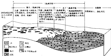
图 1 三角洲水上和水下部分各种沉积物分布特征（据 E. H. Rainwater “三角洲的地质意义”，刊于《三角洲的地质学》，休斯顿地质学会，1966）
