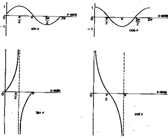
图3 某些三角函数的图形
