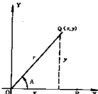
图2 标准位置的角
