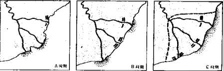
图 2 三角洲随时间外移的模式
