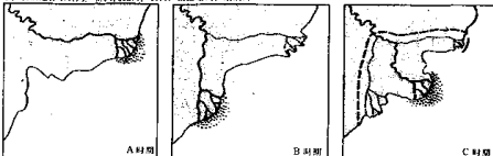
图 1 三角洲水上和水下部分各种沉积物分布特征（据 E. H. Rainwater “三角洲的地质意义”，刊于《三角洲的地质学》，休斯顿地质学会，1966）
