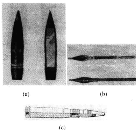
图 1.1 典型炮弹
