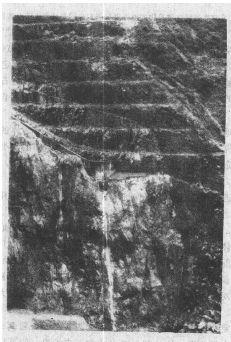
图 1-3 哥伦比亚奇沃 (Chivor) 堆石坝河岸溢洪道的挑流坎 注意左下角的道路和交通隧洞,以及挑流坎下的排水隧洞〔英格特克 (Ingetec) 公司的工程师提供的照片〕
