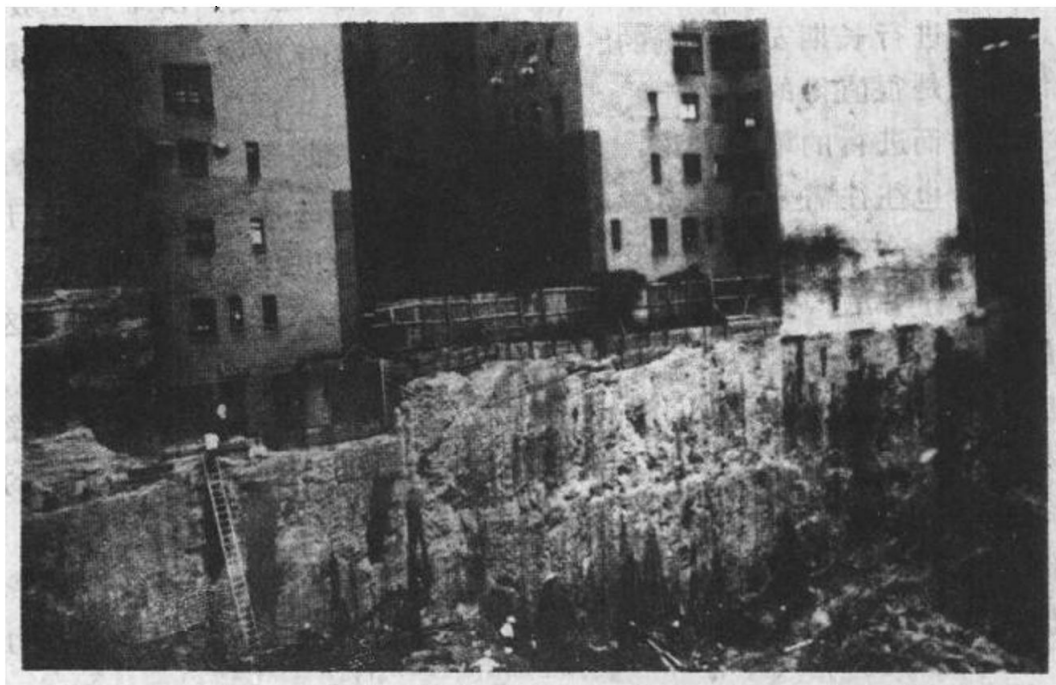
图 1-2 在非常靠近已有建筑物的地方进行岩石开挖是城市建设中常遇到的问题
