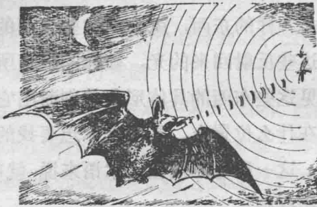
图 2 蝙蝠用超声波探测目标
