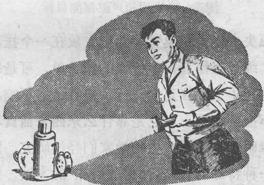
图1 光的反射使我们能看到东西
