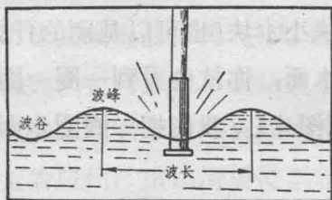
图 5 波峰、波谷和波长
