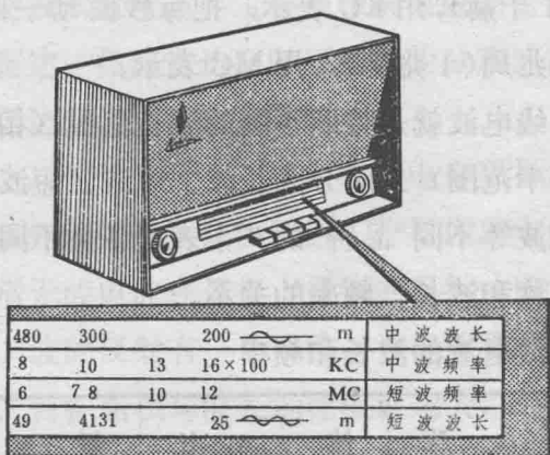
图6 频率越高，波长越短
