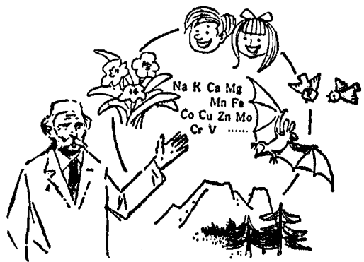
图 1 有生命物质和无生命物质都由化学元素所组成
