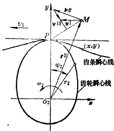
图1-3 齿条与齿轮啮合
