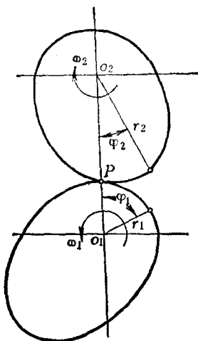
图1-2 瞬心线
