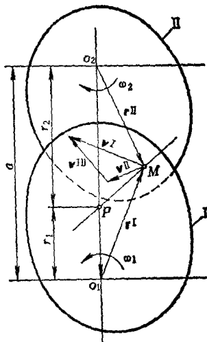
图1-1 两齿轮的相对运动
