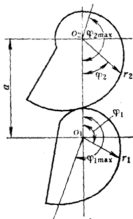
图1-4 i_{12} 随 \varphi_1 均匀变化的一对瞬心线
