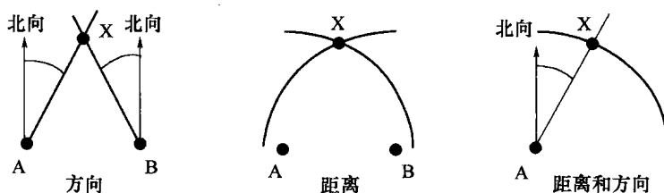
图 1.1 测量方向和距离的定位方法
