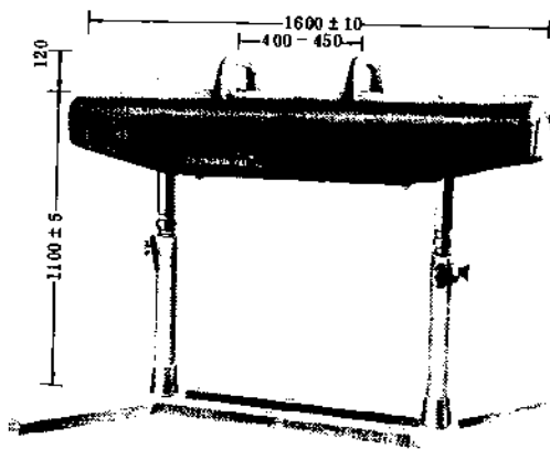
图 2 鞍马规格示意图
