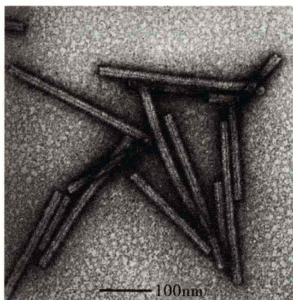
图2 烟草花叶病毒电镜照片
