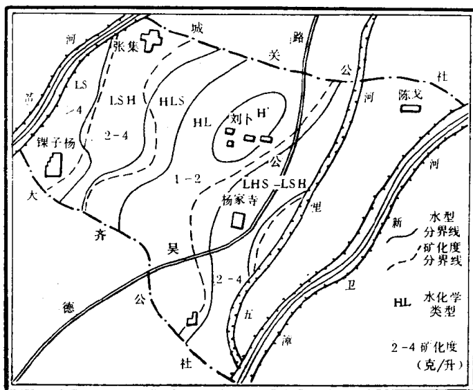
图 6 杨家寺公社浅层承压水水化学图
