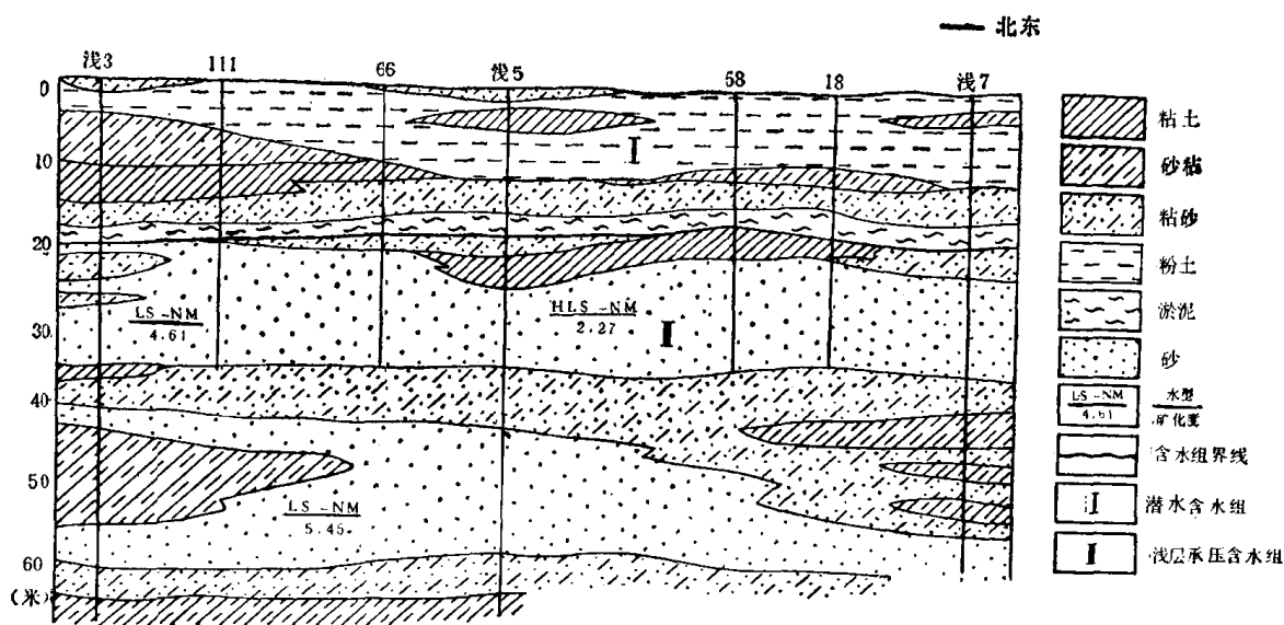
图2 杨家寺公社水文地质剖面示意图
