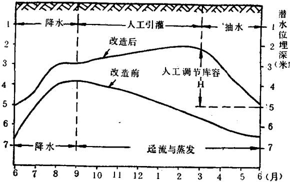
改造前后潜水动态特征对比示意图
