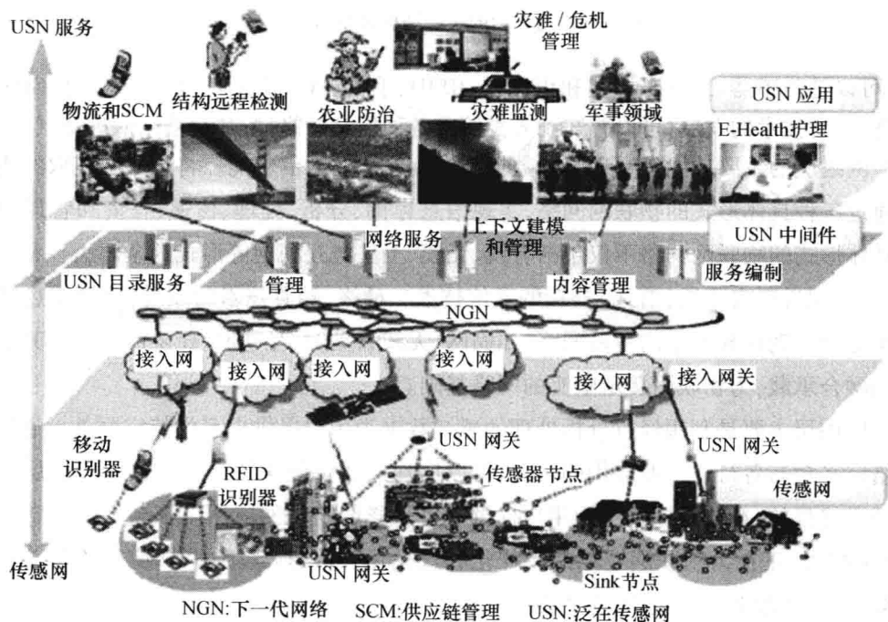
图 2-2 ITU 提出的物联网结构
