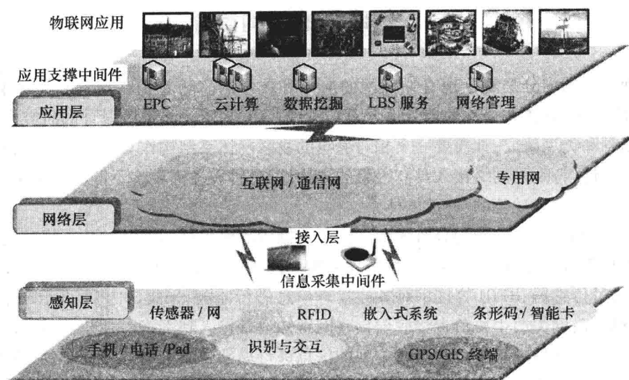
图 2-3 物联网的三层结构模型示意图
