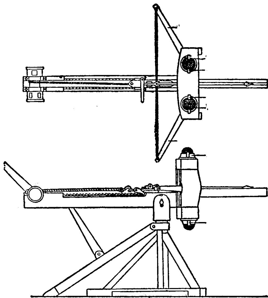
罗马弩炮
