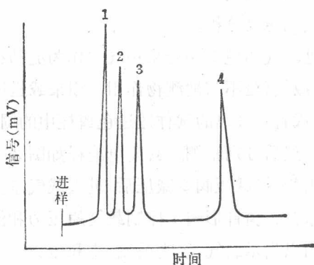
图 2-2 色谱图
