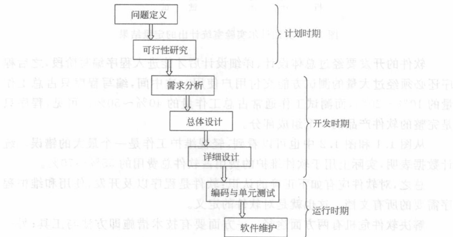
图 1.3 瀑布模型
