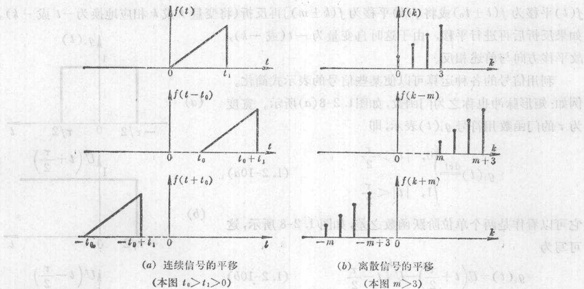
图 1.2-5 信号的平移
