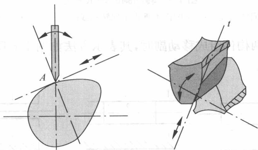
图 1-4 高副
