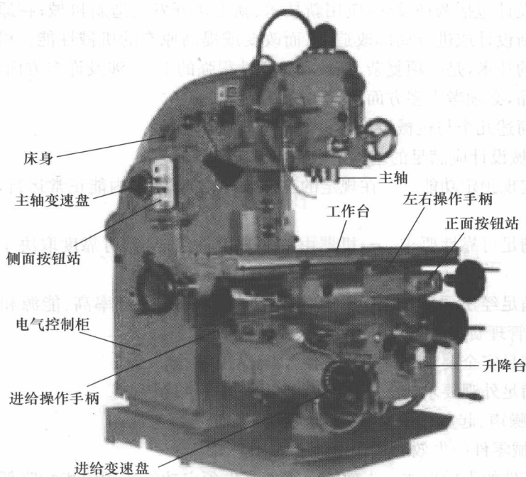
图 1-1 万能铣床
