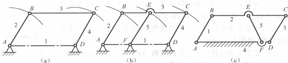
图 1-12 运动轨迹重合引入虚约束
