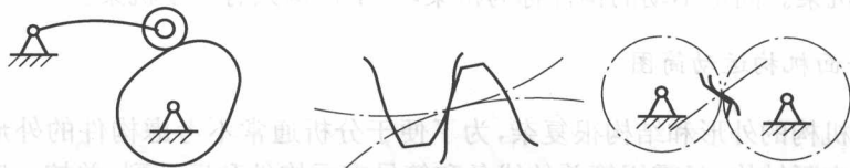
图 1-7 平面高副的表示方法
