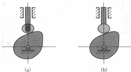
图 1-11 局部自由度
