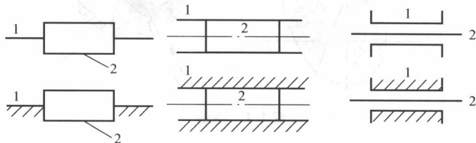
图 1-6 移动副的表示方法
