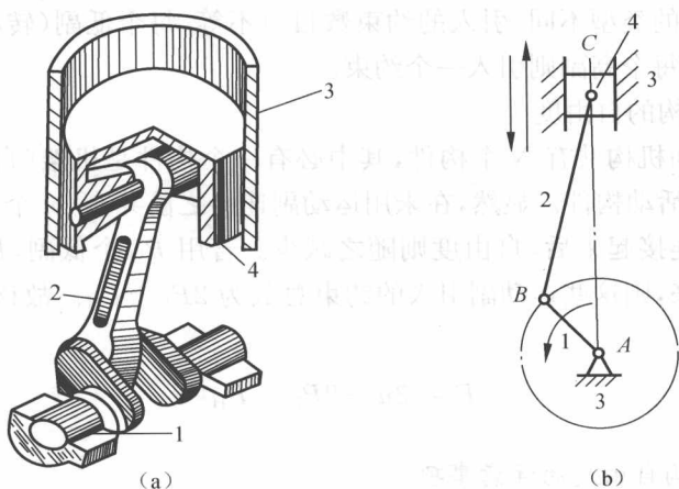
图 1-8 内燃机部分结构与机构运动简图
