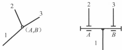
图 1-10 复合铰链
