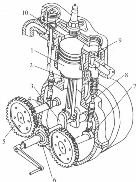
图 1-1 单缸内燃机
