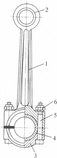
图 1-3 连杆的组成
