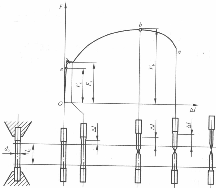
图 1-6 低碳钢的力-伸长曲线
