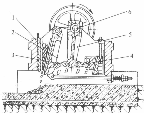
图 1-2 颚式碎矿机
