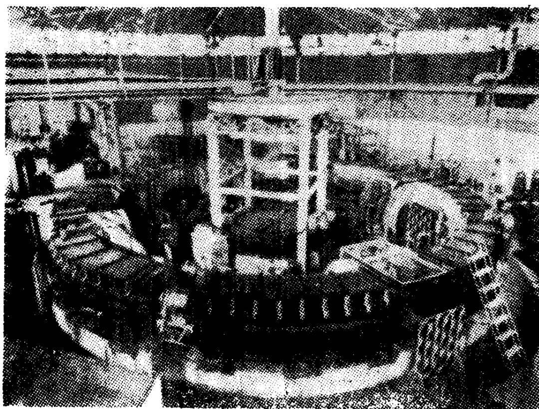
第 3 图 东京大学原子核研究所的同步加速器(见本卷 § 32.9)
