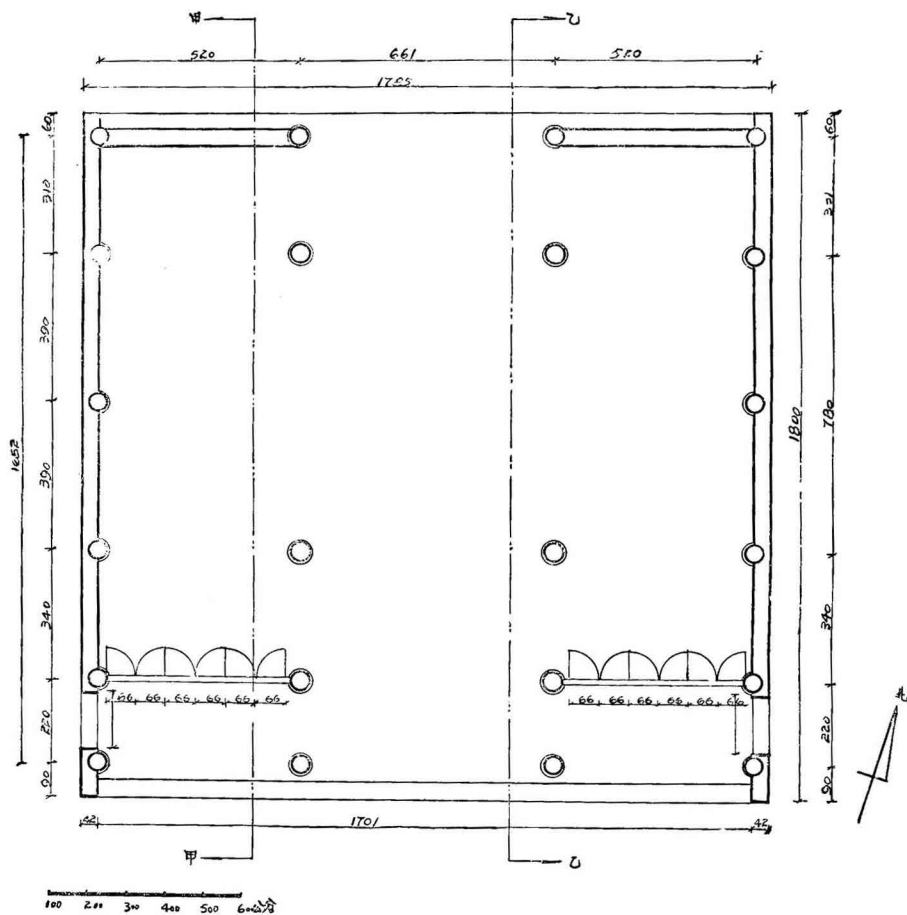
蘇州忠王府正殿平面圖(同濟大學陳從周教授繪)
