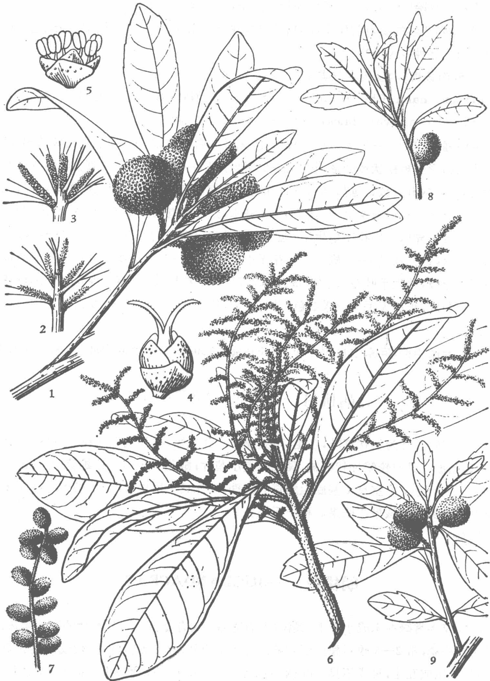
1—5. 杨梅 Myrica rubra Sieb. et Zucc.: 1.果枝; 2.部分雌花枝; 3.部分雄花枝; 4.雌花; 5. 雄花。6—7. 毛杨梅 M. esculenta Buch.-Ham.: 6.雄花枝; 7.果序。8. 青杨梅 M. adenophora Hance 果枝。9. 云南杨梅 M. nana Cheval. 果枝。(吴影萍绘)
