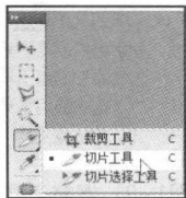
图1-5 切片工具
