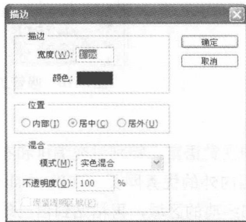
图1-7 “描边”对话框
