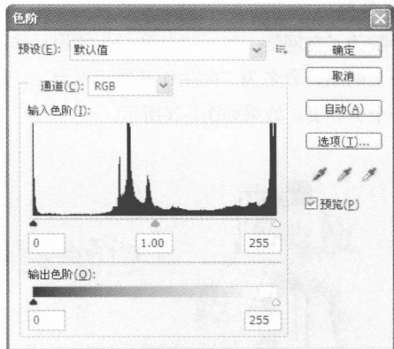
图1-25 “色阶”对话框
