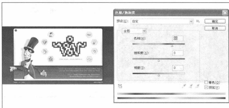
图1-18 调整“色相”后
