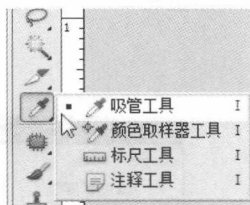
图1-10 吸管工具
