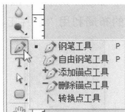
图1-9 钢笔工具
