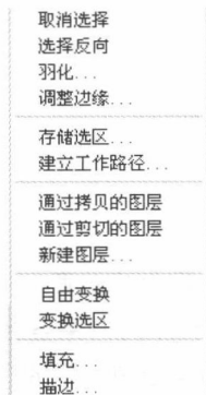
图1-6 快捷菜单
