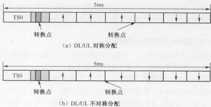
图 1-3 TD-SCDMA 时隙分配示例
