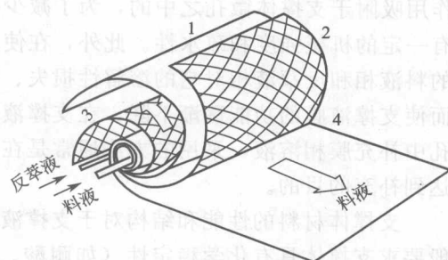
图 2-5 卷包型支撑液膜装置
