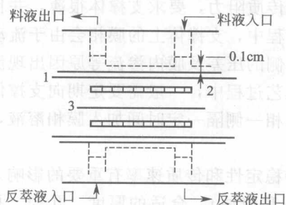
图 2-4 平板型支撑液膜装置剖面图
