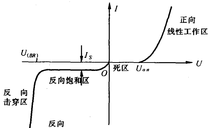
图 1-10 二极管的伏安特性
