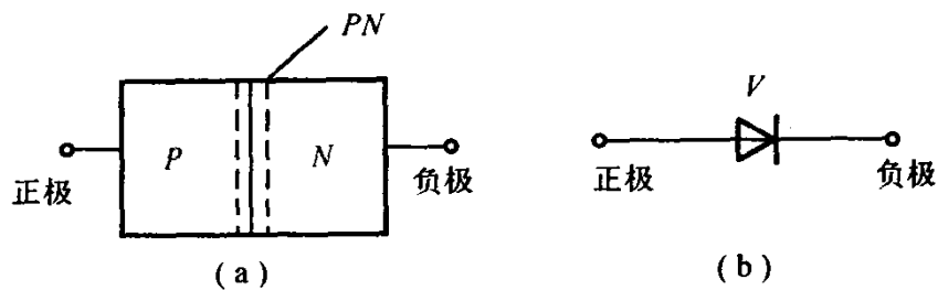
图 1-8 二极管的结构示意图与电路符号 (a)结构示意图; (b)电路符号
