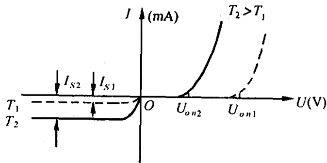
图 1-11 伏安特性曲线受温度的影响
