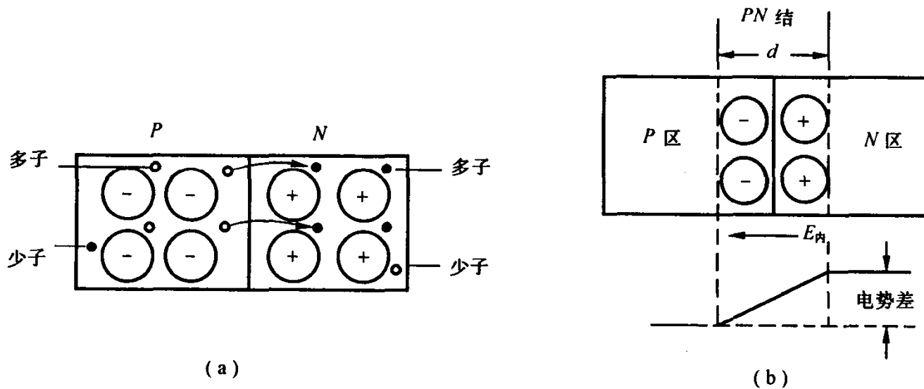
图 1-4 PN 结的形成过程 (a)多子的扩散； (b)PN 结形成
