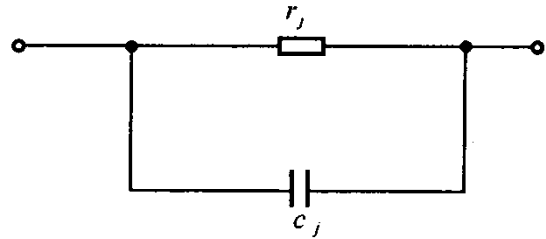
图 1-7 PN 结高频等效电路
