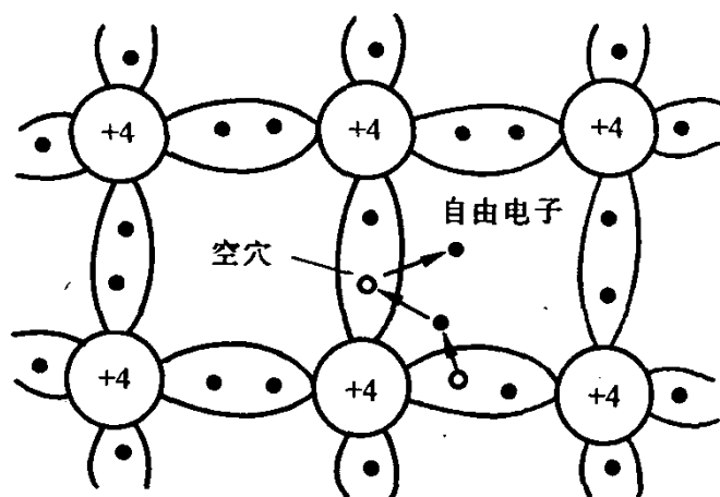
图1-1 本征半导体中的载流子
