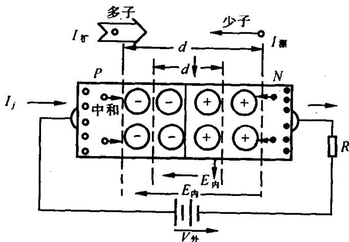
图1-5 PN结正向加压
