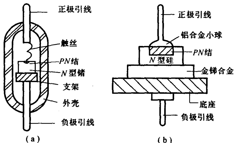
图 1-9 二极管的结构 (a)点接触型; (b)面接触型
