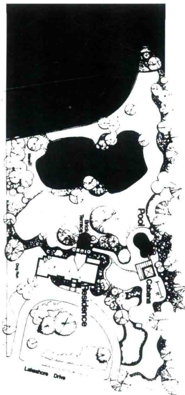
滨水别墅绿化平面图
