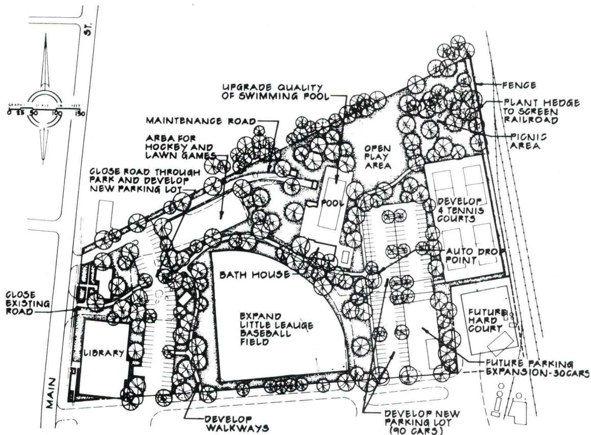
街头小型活动公园平面图
