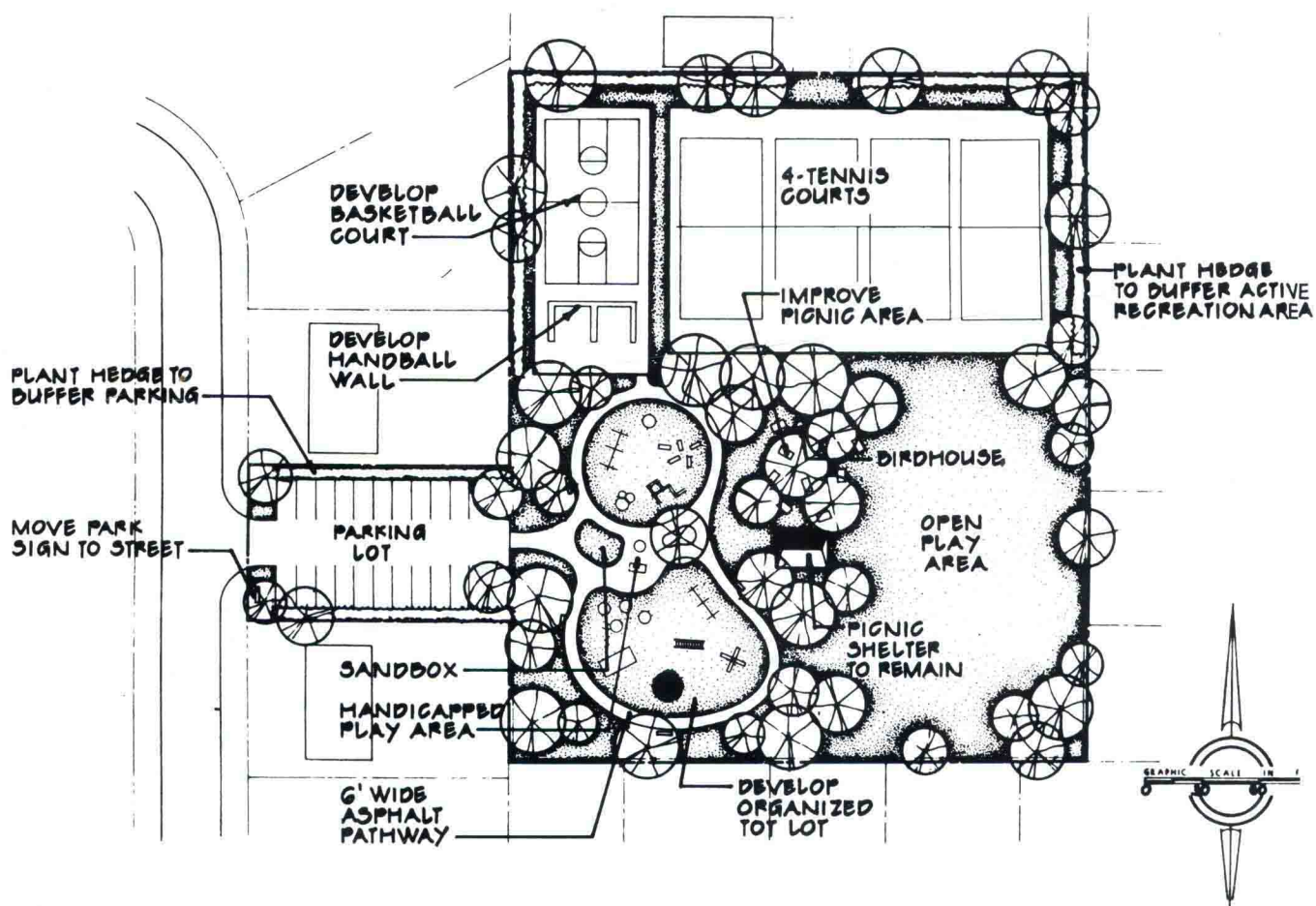
某小型活动场地规划平面图
