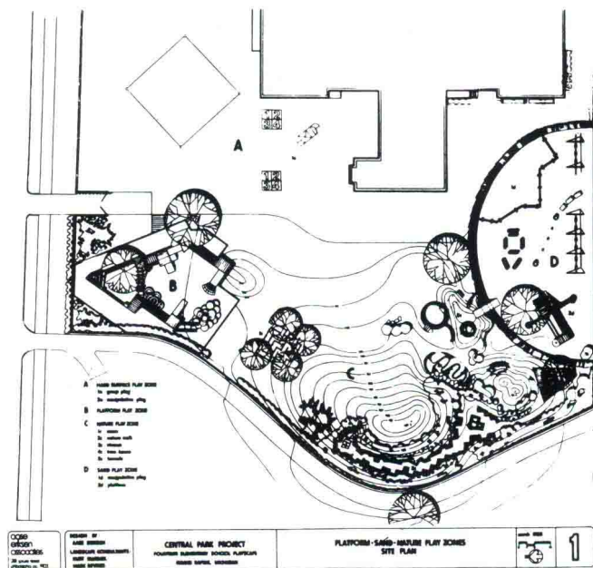
(美)某中心公园设计方案平面图
