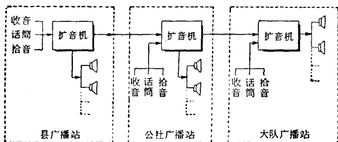
图7 农村有线广播网示意图
