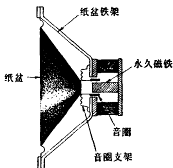
图3 动圈式喇叭的构造
