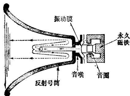
图4 高音喇叭的构造
