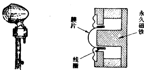
图2 动圈式话筒的外形(左)和构造(右)
