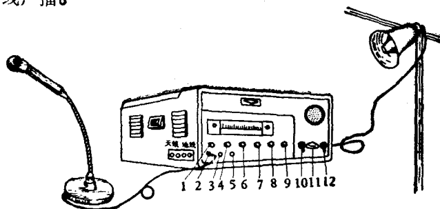
图 6 有线广播的组成
