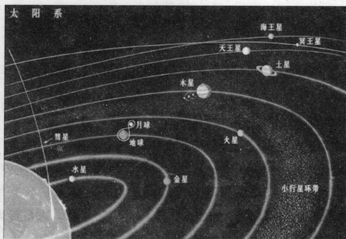
太阳系
