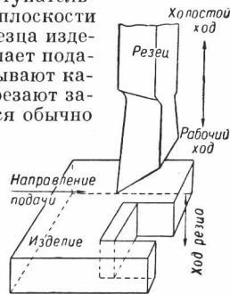
Схема процесса долбления.
