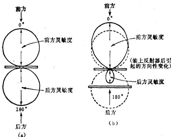
图2.9 前后比 (F/B)
