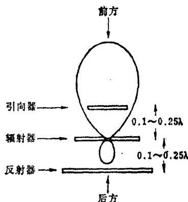
图 2.4 八木天线的基本结构
