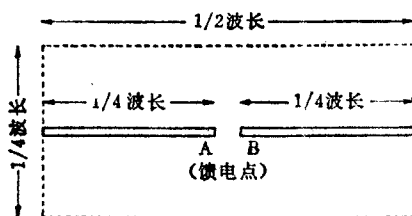
图2.1 半波长偶极子天线
