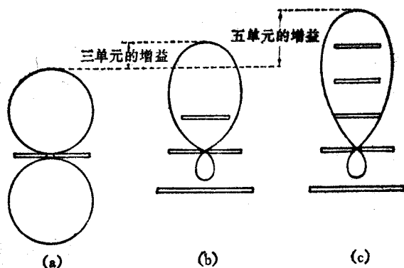
图2.7 单元数与增益
