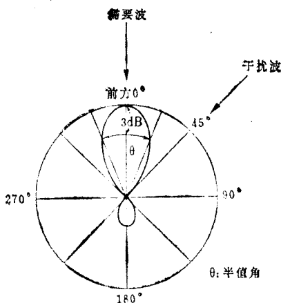
图 2.6 半值角
