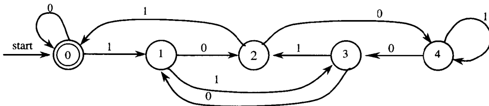
图 1.2 接受能被 5 整除的二进制数的 DFA
