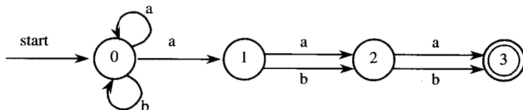
图 1.7 接受正规式 (a \mid b)^* a (a \mid b) (a \mid b) 的 NFA
