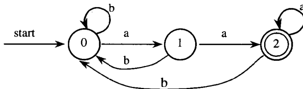
图 1.8 接收 (a \mid b)^* aa 的 DFA
