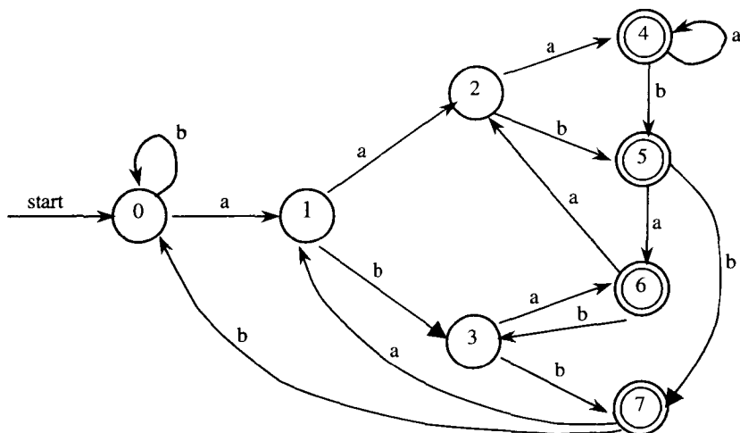
图 1.11 接收 (a \mid b)^* a (a \mid b) (a \mid b) 的 DFA
