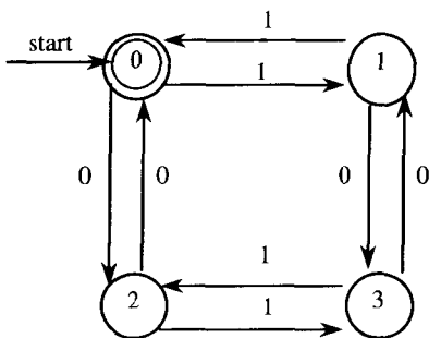
图 1.1 接受偶数个 0 和偶数个 1 的 DFA
