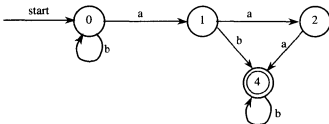
图 1.14 最简 DFA
