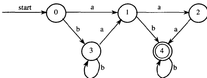
图 1.13 一个 DFA
