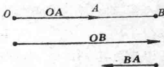
图 1-1-5 直线运动中位移和路程的区别
