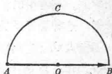
图 1-1-3 位移与路程的区别
