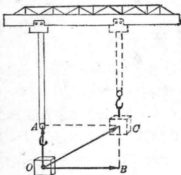
图 1-1-7 用平行四边形合成矢量
