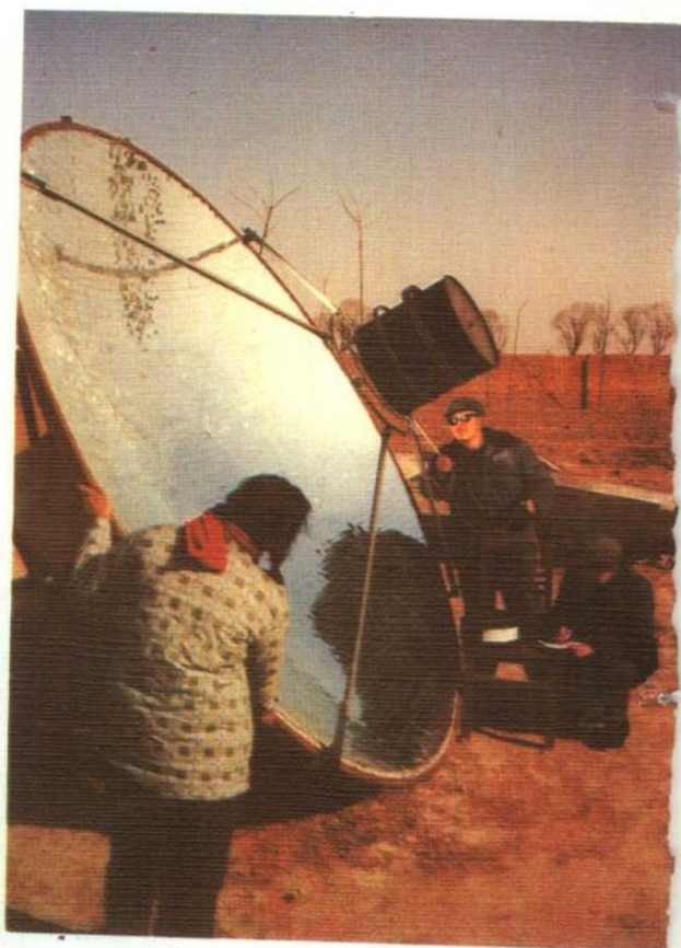
虞城县和郑州工学院合作研究 太阳能贮存装置
