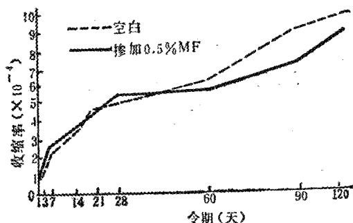
图 4 MF 对普通水泥砂浆干缩影响
