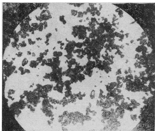
图 2 未掺 MF (水泥粒子的扩散效应〈显微照相×110〉)
