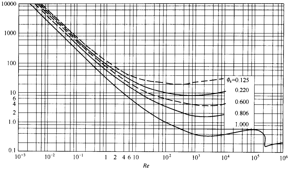
图 1-1-2 \zeta-Re 的关系曲线
