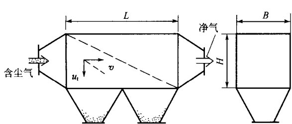
图 1-1-3 沉降室中尘粒的运动
