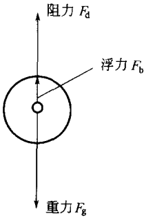
图 1-1-1 沉降尘粒的受力情况
