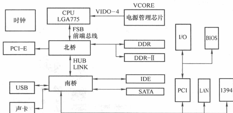
图 1-2 主板各模块组成
