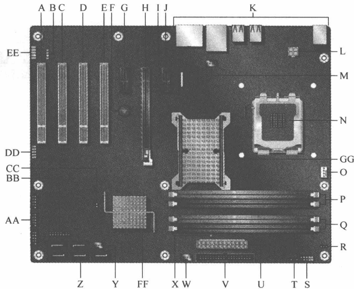
图 1-1 主板布局图
