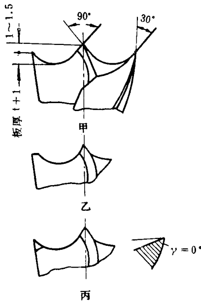
图 II-1-6 薄板钻
