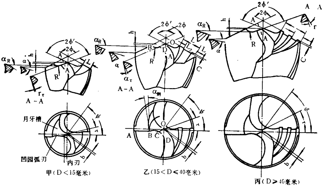
图 II-1-3 标准群钻
