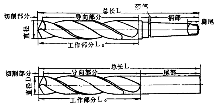
图Ⅱ-1-1 麻花钻的构造
