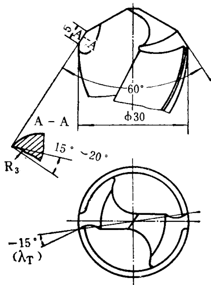
图Ⅱ-1-7 加工钢的精孔扩钻
