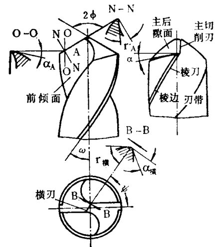
图Ⅱ-1-2 麻花钻的切削角度
