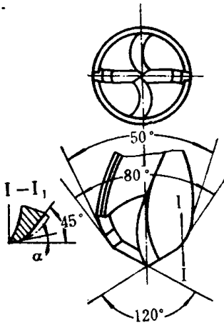
图 II-1-4 铸铁钻头的结构
