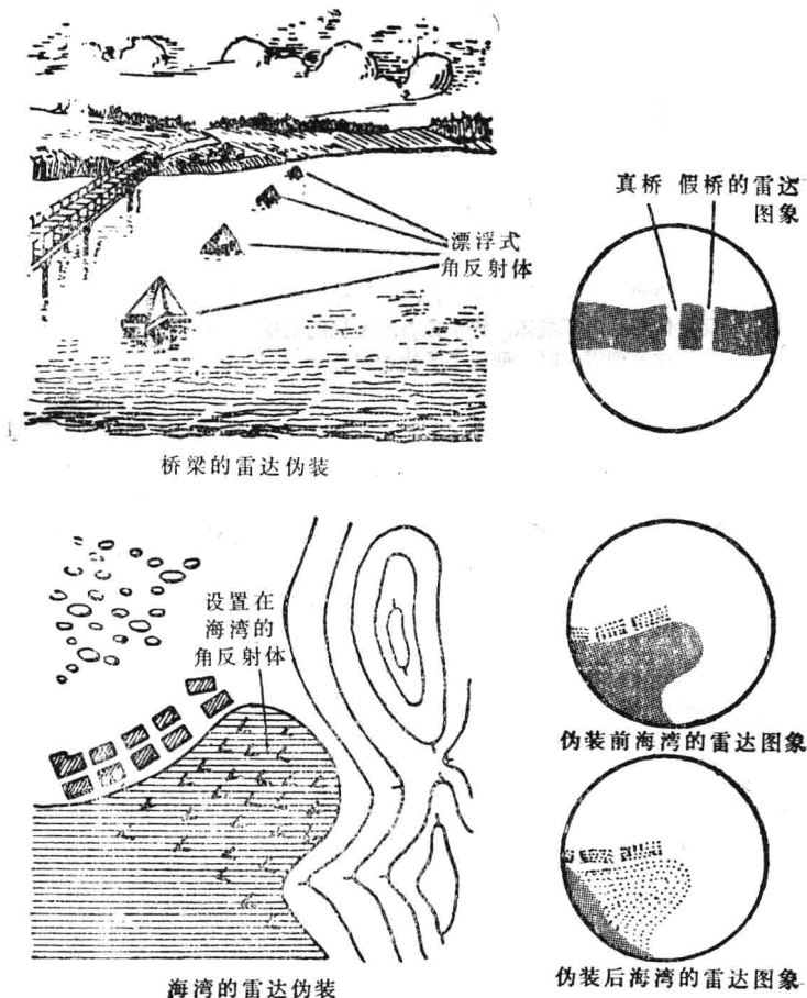
图3 应用角反射器的效果
