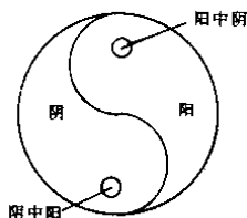
图 1.2 太极图
