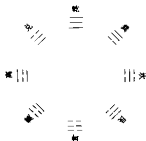
图 1.8 先天八卦图
