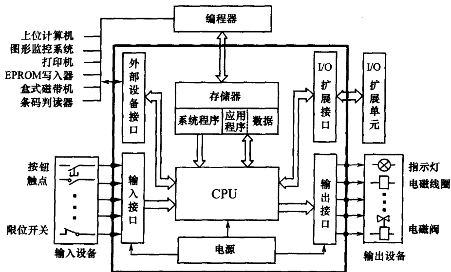
图 2-1 PLC 硬件系统结构图
