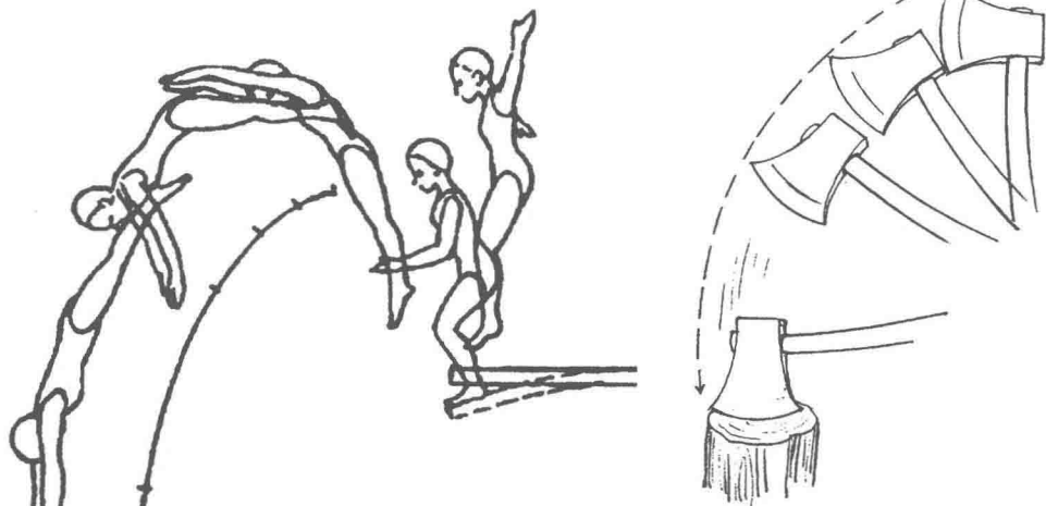
图1-2-5 斧子砍下的加速运动 斧子砍下因外力作用便产生了加速运动。
