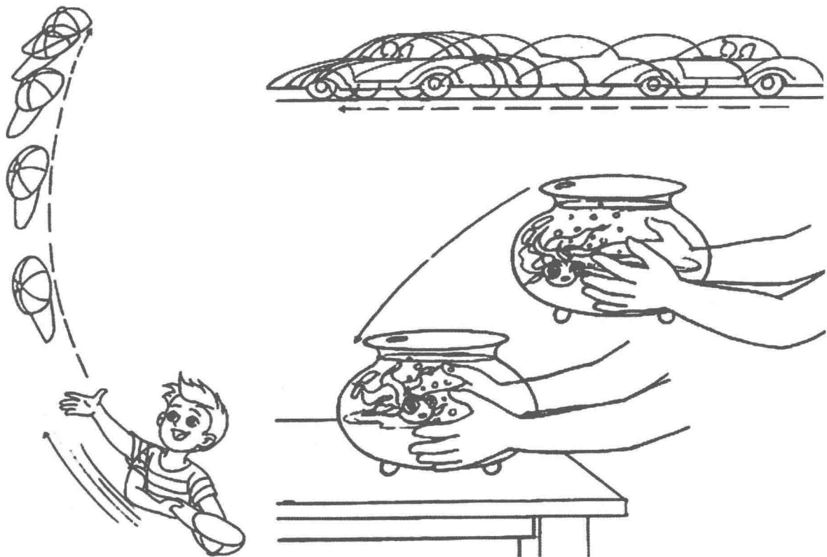
图1-2-7 减速运动
