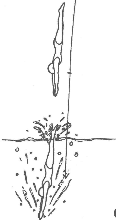
图1-2-4 运动员高台跳水的加速运动 跳水运动员在高空下坠的时候由于地心引力的作用，在下落的过程中速度越来越快，产生了加速运动。
