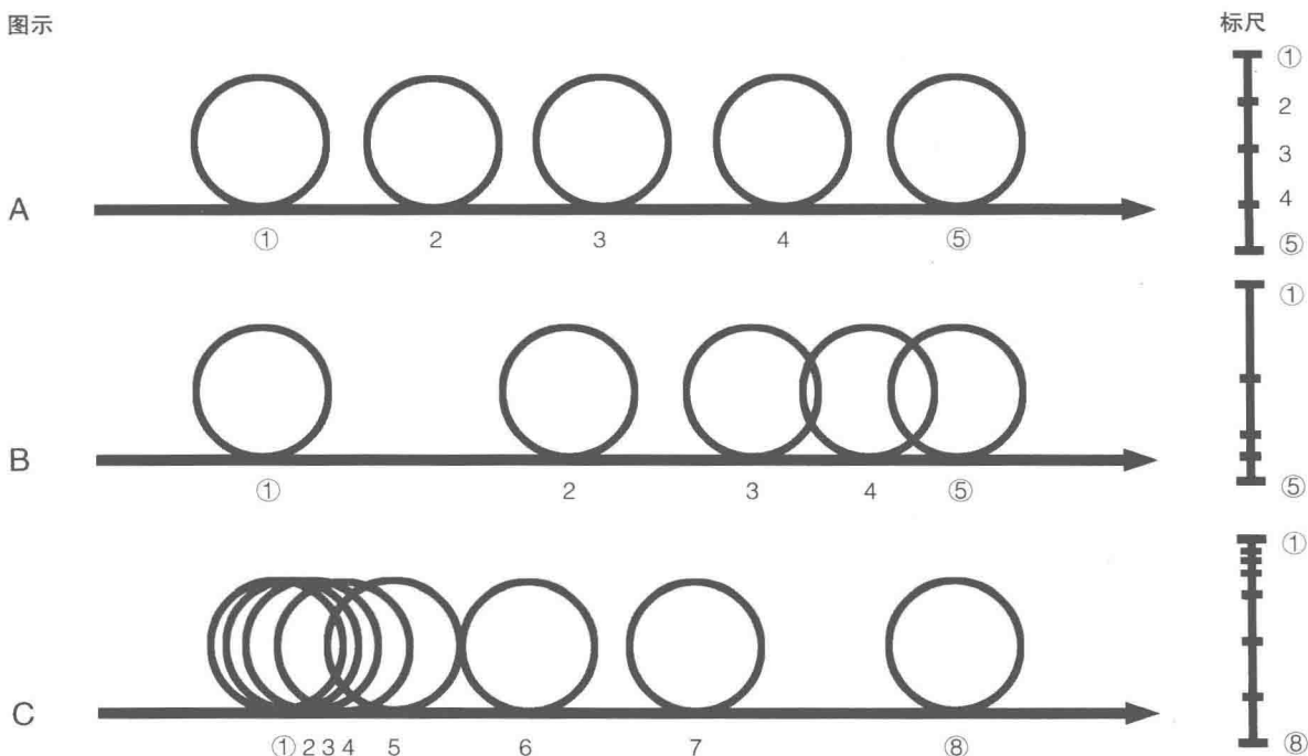
图1-2-3 球的运动速度和位置变化
