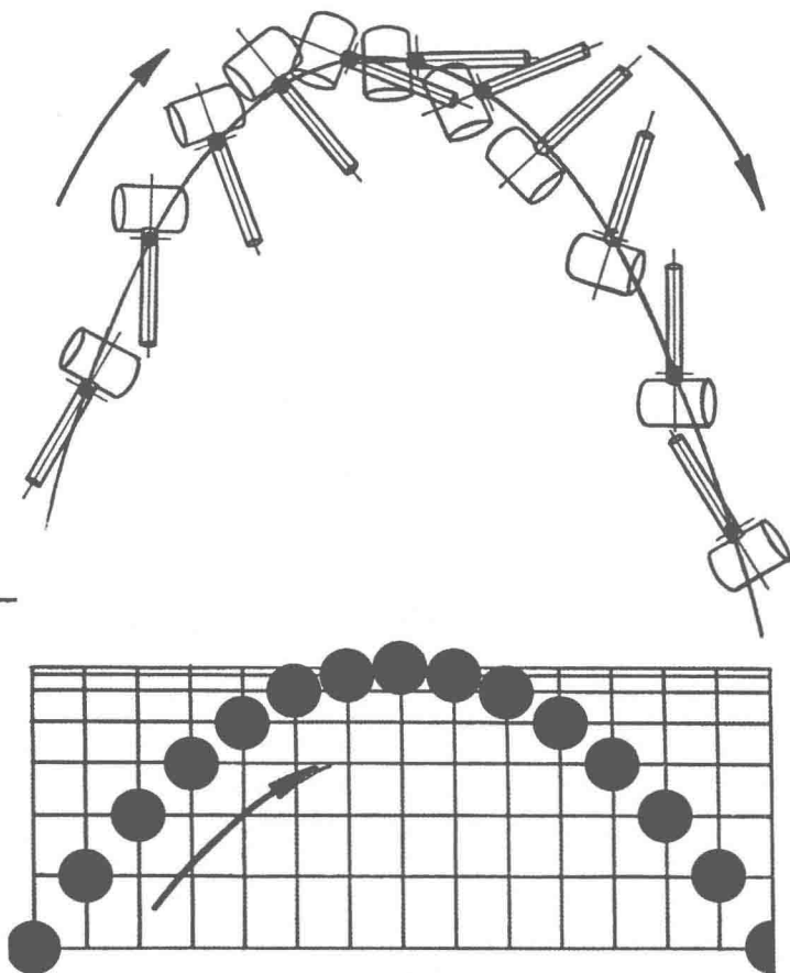
图1-2-6 抛物运动 由于受各种力的作用，抛物运动是一个加减速运动。上图中锤子被由左向右抛出。我们可以看到每张动画锤子的距离变化，锤子的运动是由快到慢然后再快。锤子的运动变化同下图向上抛的小球的抛物运动。
