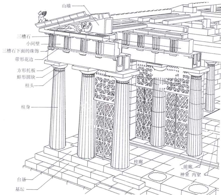
图 1-2 古希腊时期建筑装饰
