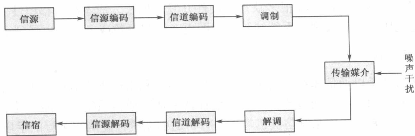
图 1-1 点对点数字通信系统
